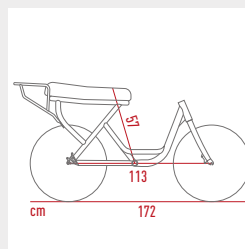
Dimensioni e-bike
